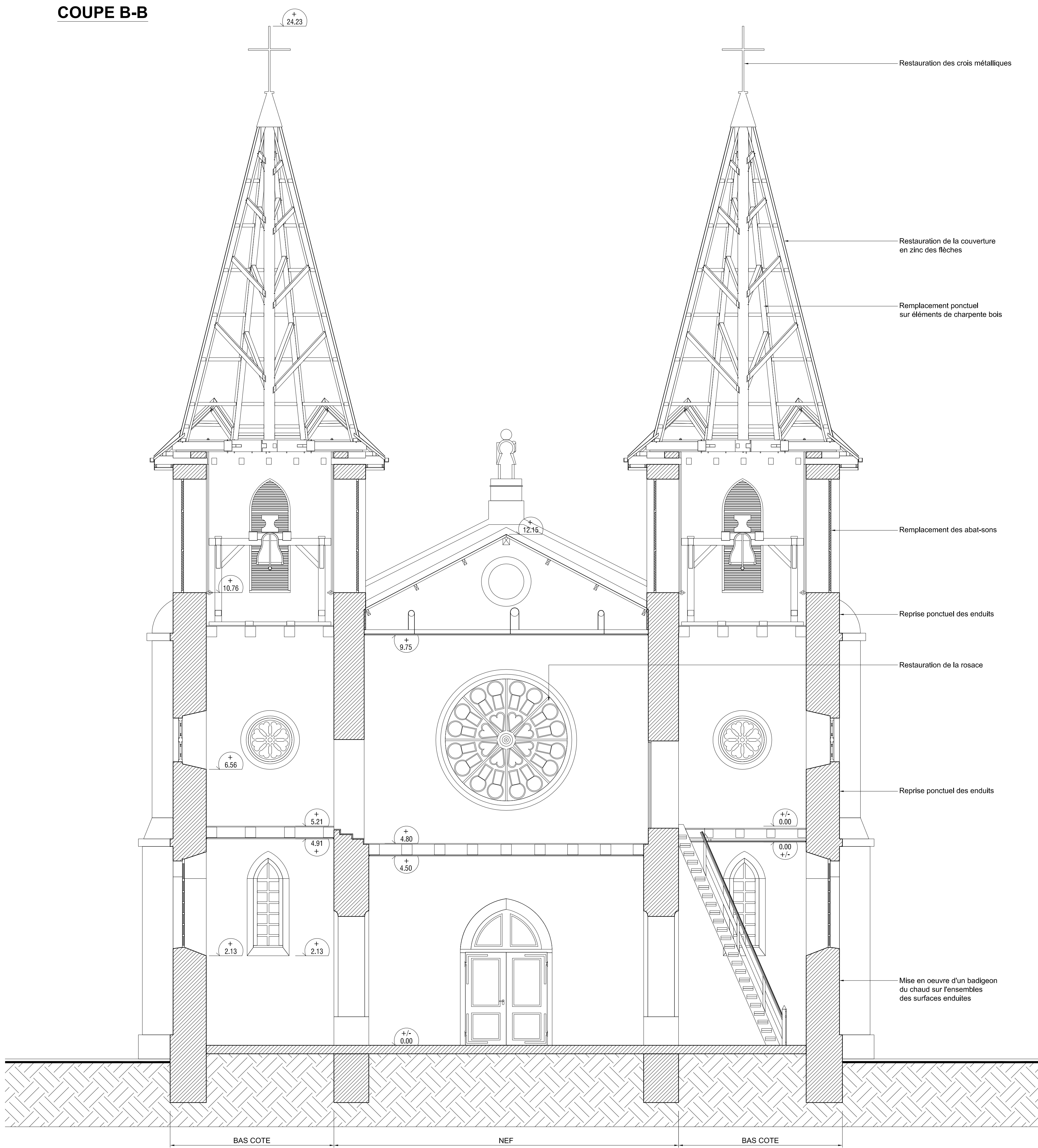
COUPE B-B
